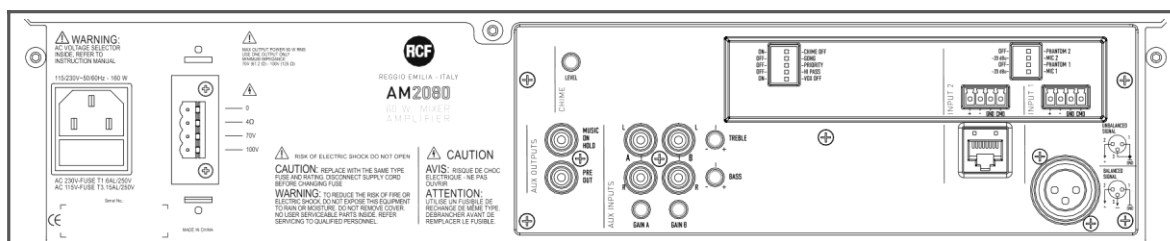
Panel tylny
